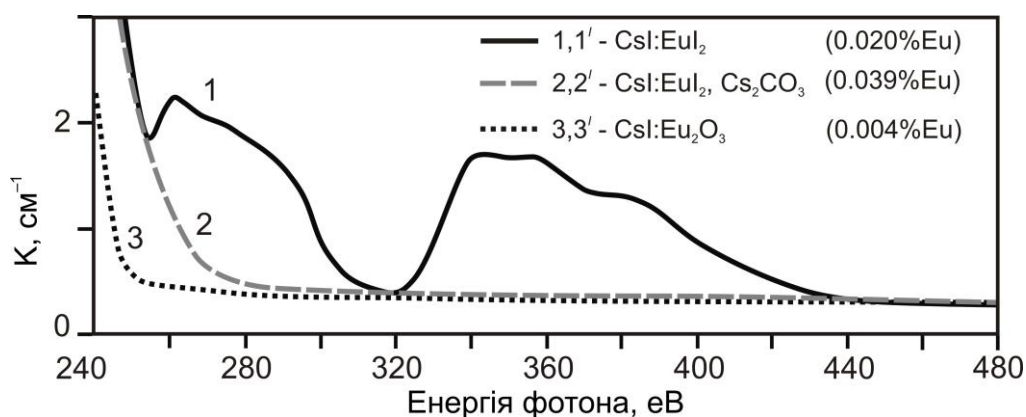
Рис. 1. Спектри поглинання (1-3) кристалів CsI:Eu, активованих \text{EuI}_2 (1,2,) і \text{Eu}_2\text{O}_3 (3) з домішкою \text{Cs}_2\text{CO}_3 (2). T=295 K
