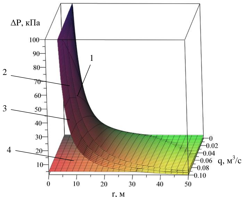
Рисунок 5. Величини розрахункового надлишкового тиску вибуху в залежності від відстані від центру вибуху ( r ) та витрати газу ( q ): 1 - \Delta P(\tau_3=300 \text{ с}) , 2 - \Delta P(\tau_2=120 \text{ с}) , 3 - \Delta P(\tau_1=10 \text{ с}) , 4 - \Delta P=5 \text{ кПа}
