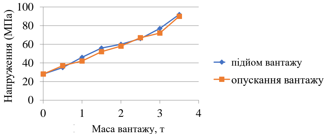
Рис. 6. Тарувальна крива
