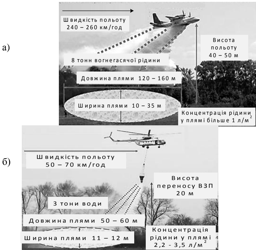
Рисунок 1 – Режим польоту при зливі вогнегасної рідини та параметри утвореної плями (а – з літака, б – з водозливного пристрою гелікоптера)
