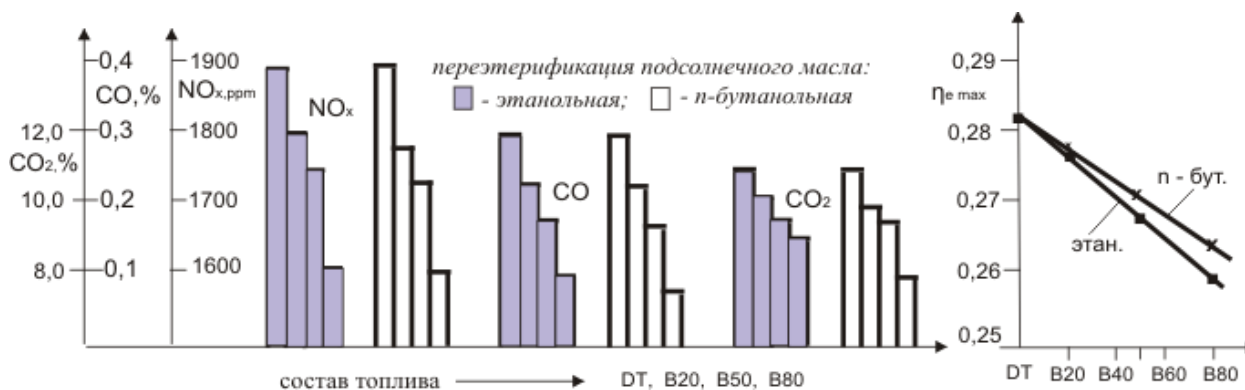
Рис. 2. Усредненные значения выбросов вредных веществ с ОГ и максимальные значения КПД двигателя 4СН 7,9/7,5 (VW)
