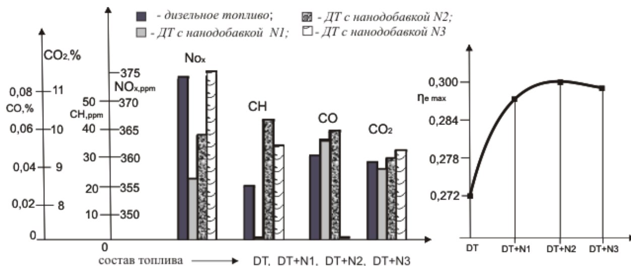
Рис.4. Влияние концентрации наночастиц в ДТ на показатели токсичности и максимального КПД дизеля 1С 8,5/11 (режим N_e = 3 \text{ кВт} , n = 1300 \text{ мин}^{-1} )
