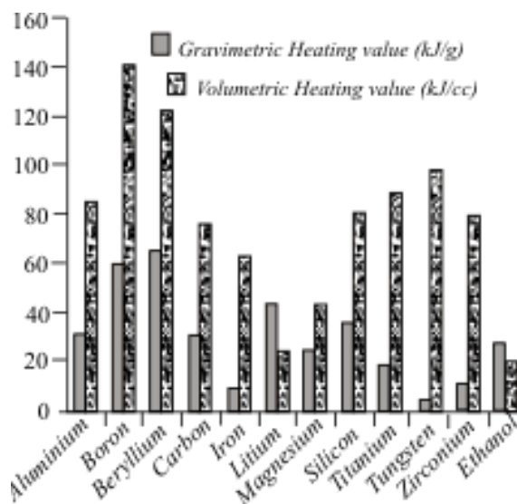
Рис. 3. Гравиметрическая и объемная теплота сгорания некоторых металлов и этанола
