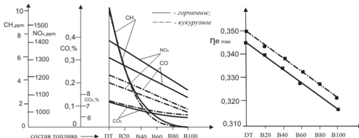
Рис. 1. Усредненные значения выбросов вредных веществ с ОГ и максимальные значения КПД двигателя 2С10,5/12
