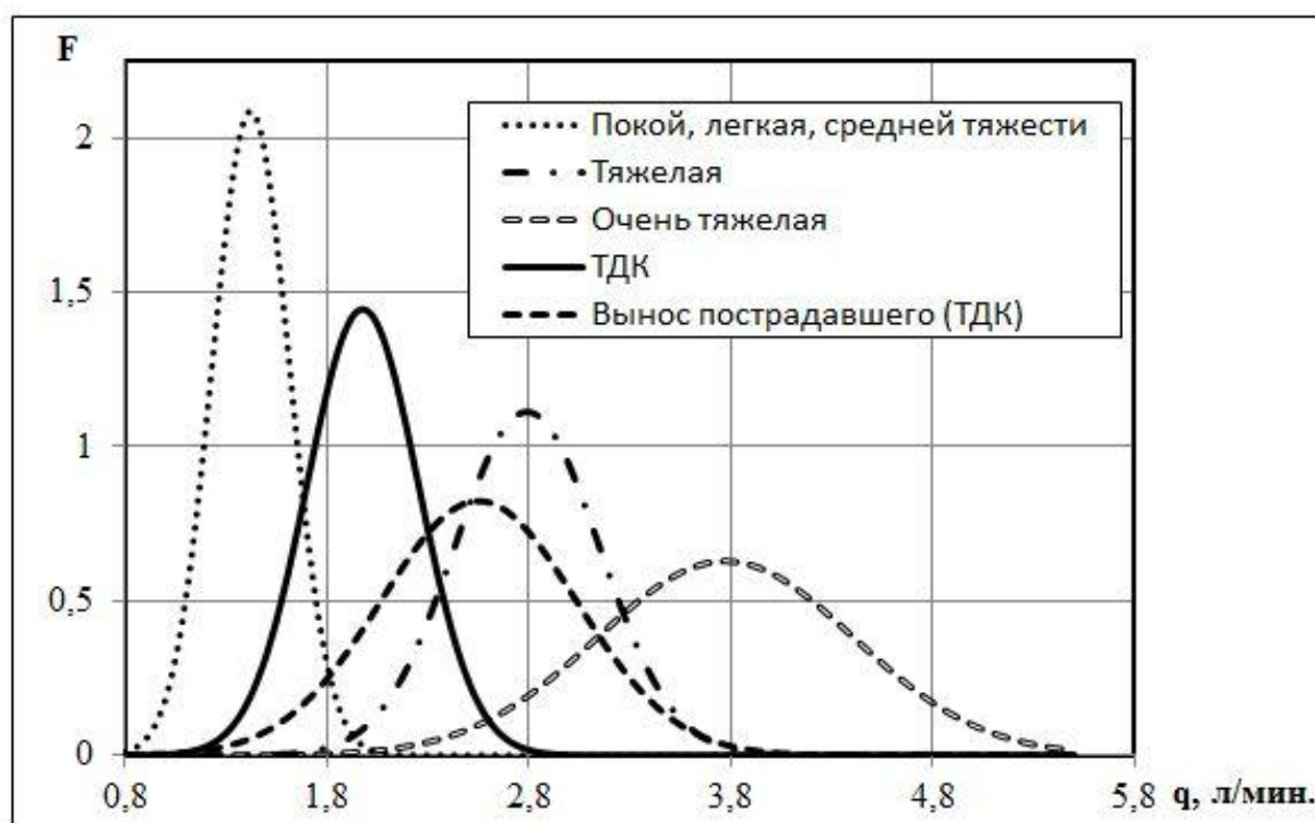
Рисунок 1 - Функции распределения расхода кислорода в РДА
