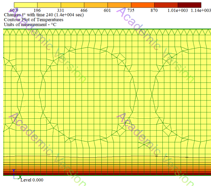
Рис. 8. Ізополя температур
