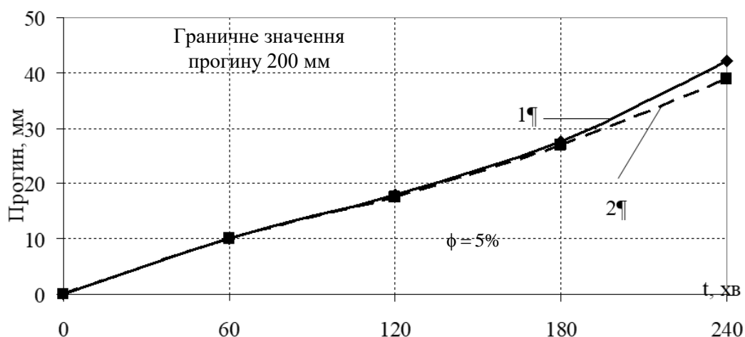
Рис. 11. Прогин залізобетонного вогнезахищеного перекриття по середині прольоту при стандартному температурному режимі пожежі: 1 – експеримент; 2 – розрахунок в програмному комплексі «ЛІРА-САПР»
