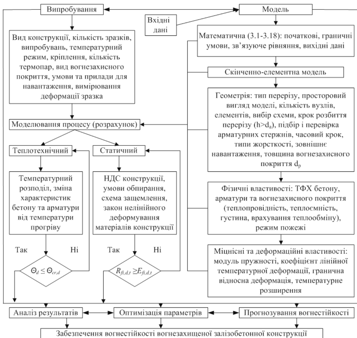
Рис. 2. Керуючий алгоритм та процедура реалізації розрахунково-експериментального методу оцінювання вогнестійкості вогнезахисних залізобетонних конструкцій
