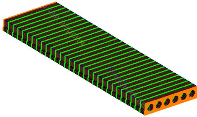
Рис. 9. Комп'ютерна модель напружено-деформованого стану вогнезахищеного залізобетонного перекриття
