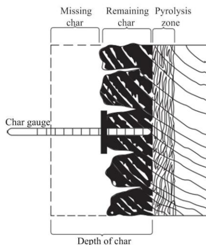
Рис. 2. Вимірювання глибини [7]
