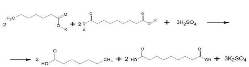
Рисунок 1. Технологія отримання азелаїнової кислоти
