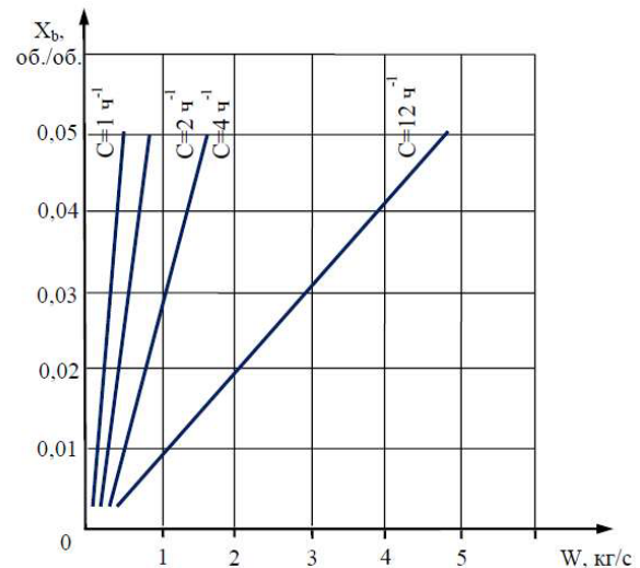
Рисунок 4 – Залежність стаціонарної концентрації X_b бензину у приміщенні від масової швидкості W витоку бензину для різної кратності повітрообміну C
