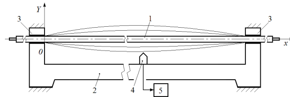
Рисунок 1. Стенд перевірочний:
