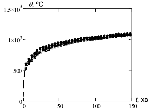
Рис. 3.3 Показники термопар у камері печі під час випробування зразків фрагментів сталевих стержнів:
