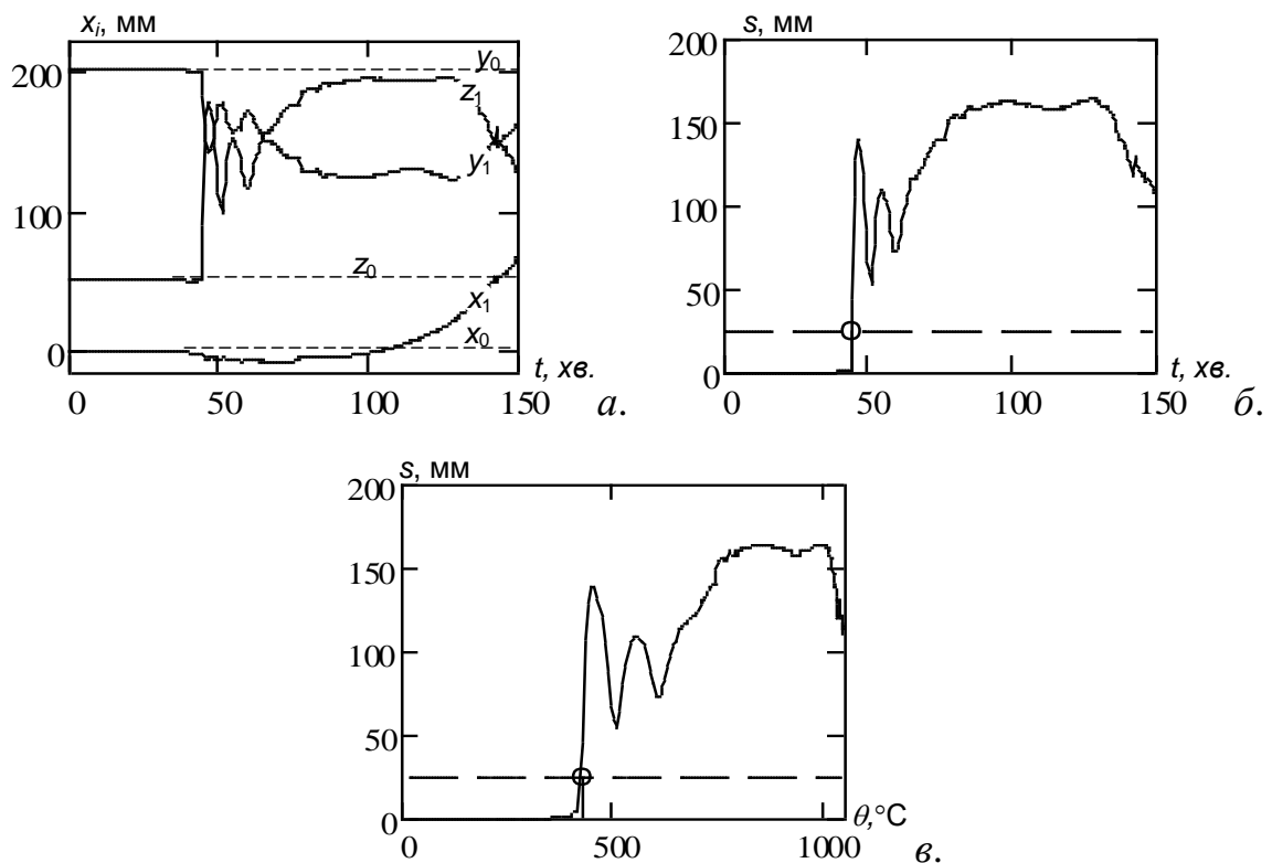
Рис. 4.20 Графіки зміни величини максимального зазору за координатами (а); графік нарощування максимального зазору, залежно від часу пожежі (б); графік нарощування максимального зазору, залежно від температури нагріву балки (в)
