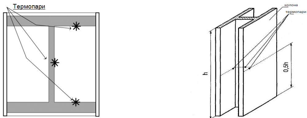
Рис. 2.7 Схема розміщення термопар на зразках сталевій колони з коробчастим перерізом
