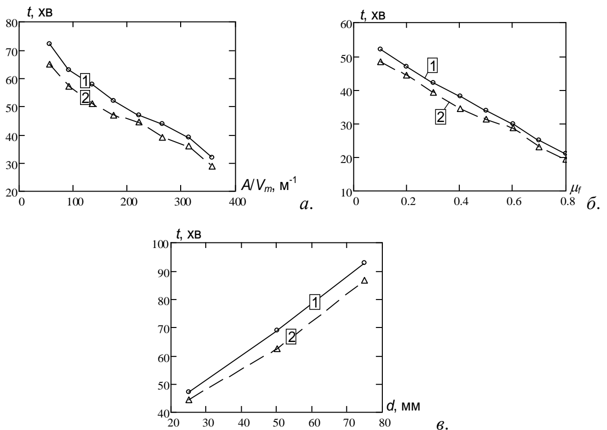
Рис. 5.5 Графіки залежності межі вогнестійкості сталеві балки з вогнезахисним мінераловатним облицюванням (1) та часу настання відшарування вогнезахисного мінераловатного облицювання (2): а – від величини коефіцієнта перерізу балки; б – від рівня прикладеного навантаження; в – від товщини вогнезахисного мінераловатного облицювання.
