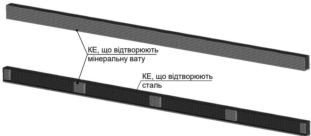
Рис. 4.12 Кінцево-елементна схема сталеві балки з вогнезахисним облицюванням із мінеральної вати
