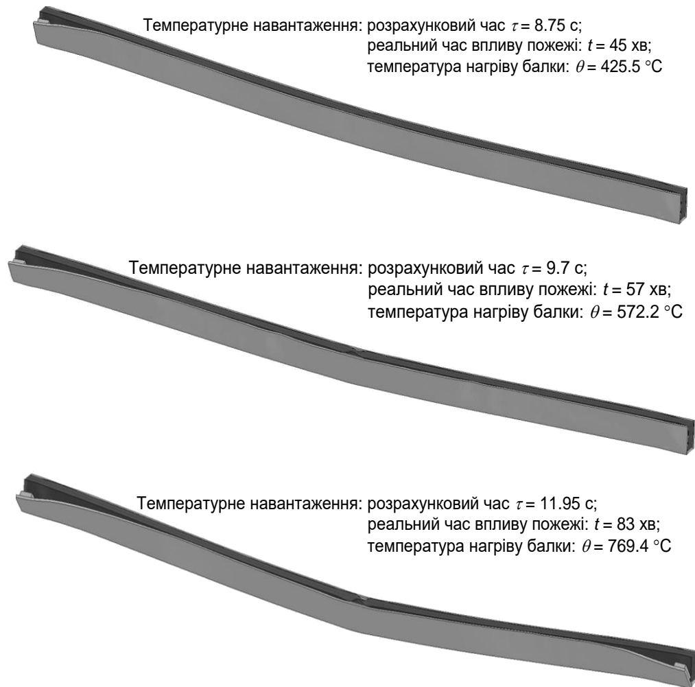
Рис. 4.19 Положення та геометрична форма облицювання в різні моменти впливу стандартного температурного режиму пожежі
