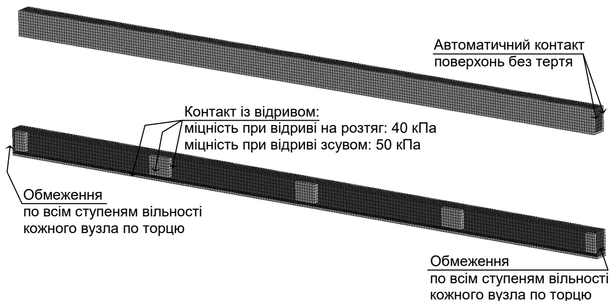
Рис. 4.13 Схема контактної взаємодії між елементами сталеві балки з вогнезахисним облицюванням із мінеральної вати
