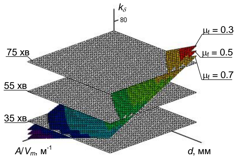
Рис. 5.6 Поверхні залежності часу відшарування вогнезахисного мінераловатного облицювання для визначення межі вогнестійкості сталевих балок для різних значень діючого навантаження
