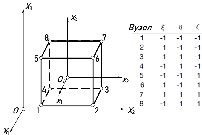
Рис. 4.6 Геометрія кінцевого елемента гексаедричного кінцевого елемента типу SOLID із вісьма вузлами
