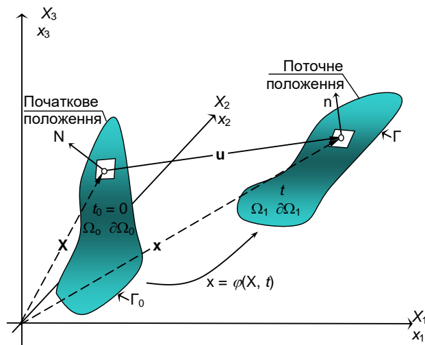
Рис. 4.3 Початковий деформований стан і поточний деформований стан твердого тіла
