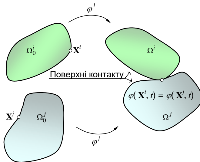
Рис. 4.4 Схема контактної взаємодії двох твердих деформованих тіл
