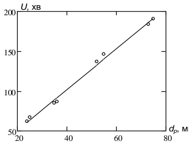
Рис. 3.6 Крива часу досягнення критичної температури 500 °С, залежно від товщини вогнезахисного облицювання
