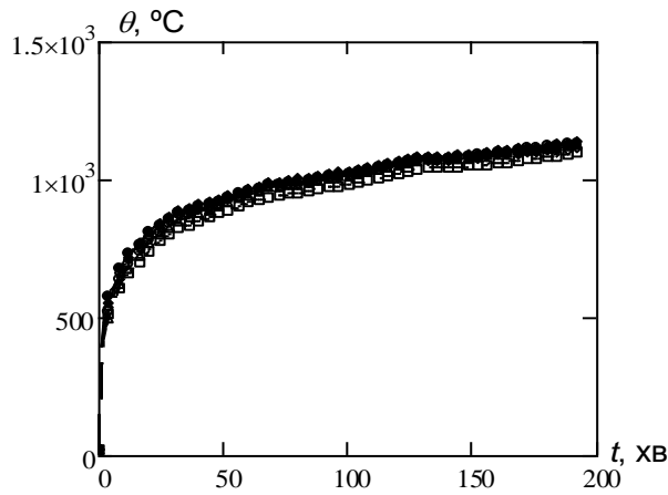
Рис. 3.3 Показники термопар у камері печі під час випробування зразків фрагментів сталевих стержнів:
