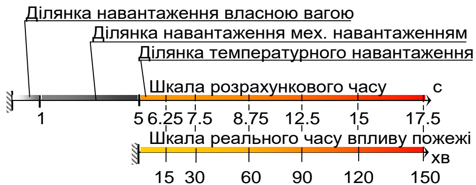
Рис. 4.15 Зіставлення шкал розрахункового часу та реального часу впливу пожежі
