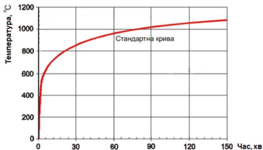
Рис. 1.3 Графік температура-час стандартного температурного режиму (відношення зростання температури до часу)
