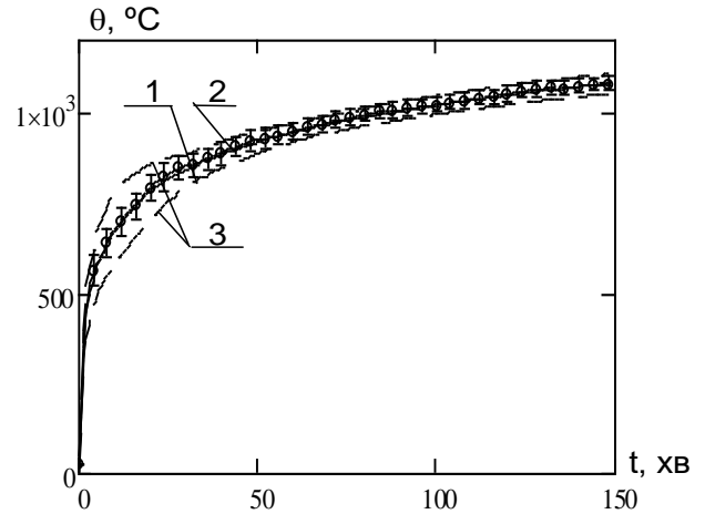
Рис. 3.4 Температурний режим випробувань у печі: 1 – середня температура в печі; 2 – стандартна температурна крива; 3 – допустимі відхилення температурного режиму.
