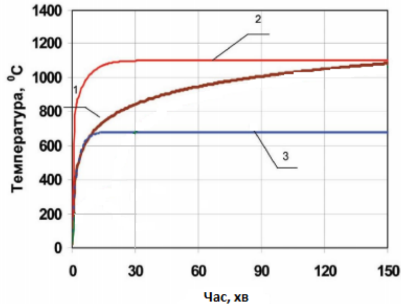
Рис. 1.5 Графік кривих температура-час номінальних температурних режимів: 1 – крива стандартної пожежі; 2 – крива вуглеводневої пожежі; 3 – крива зовнішньої пожежі
