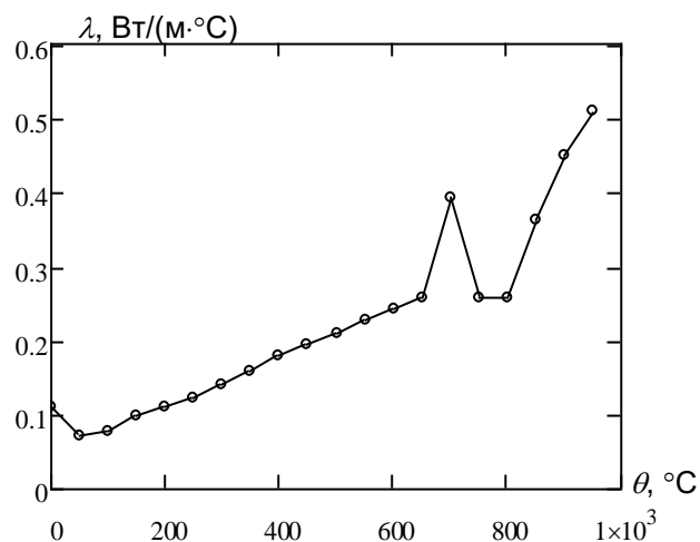
Рис. 3.13 Залежність усередненого значення коефіцієнта теплопровідності від температури зразків фрагментів сталевих стержнів із вогнезахисним облицюванням
