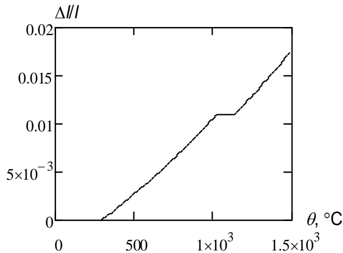
Рис. 4.8 Залежність температурної деформації сталі від температури
