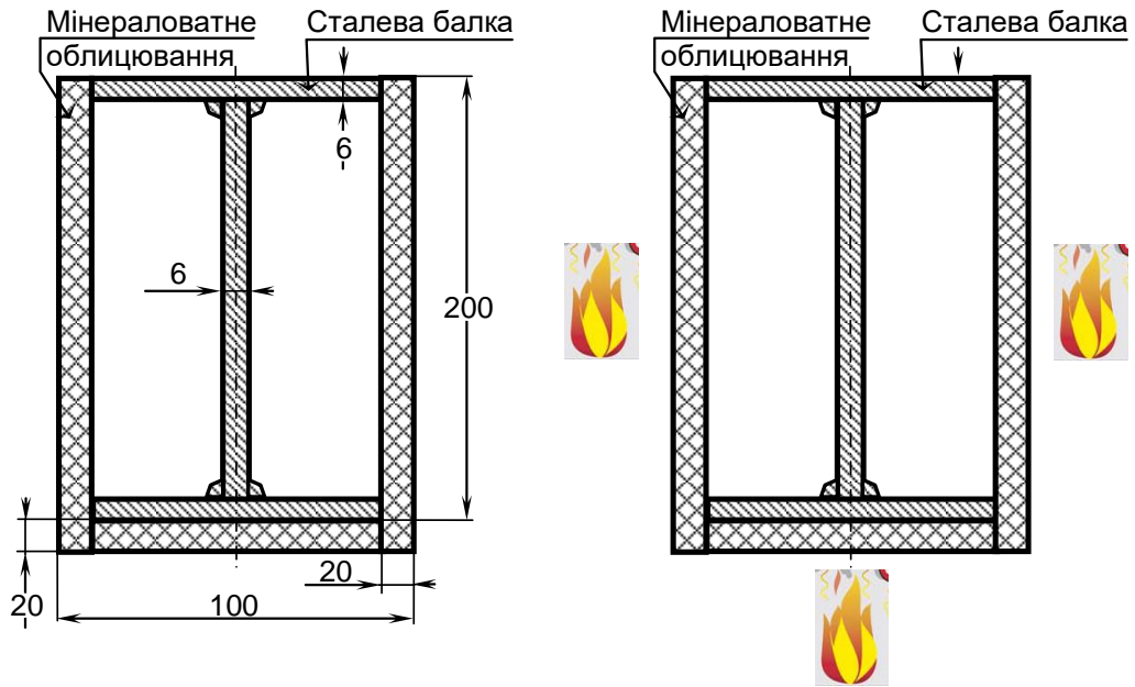
Рис. 4.1 Геометрична схема перерізу сталевієї балки з мінераловатним вогнезахисним облицюванням (а) та схема теплового впливу пожежі на переріз балки (б)
