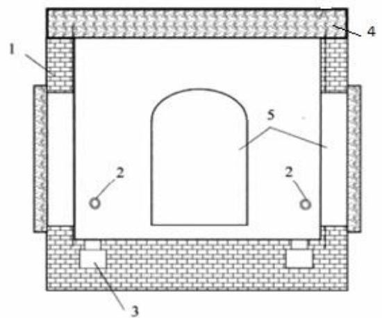
Рис. 2.1 Загальний вигляд та схема вогневої печі: 1 – корпус печі; 2 – пальники; 3 – канали видалення продуктів згорання; 4 – кришка печі; 5 – люки з дверима
