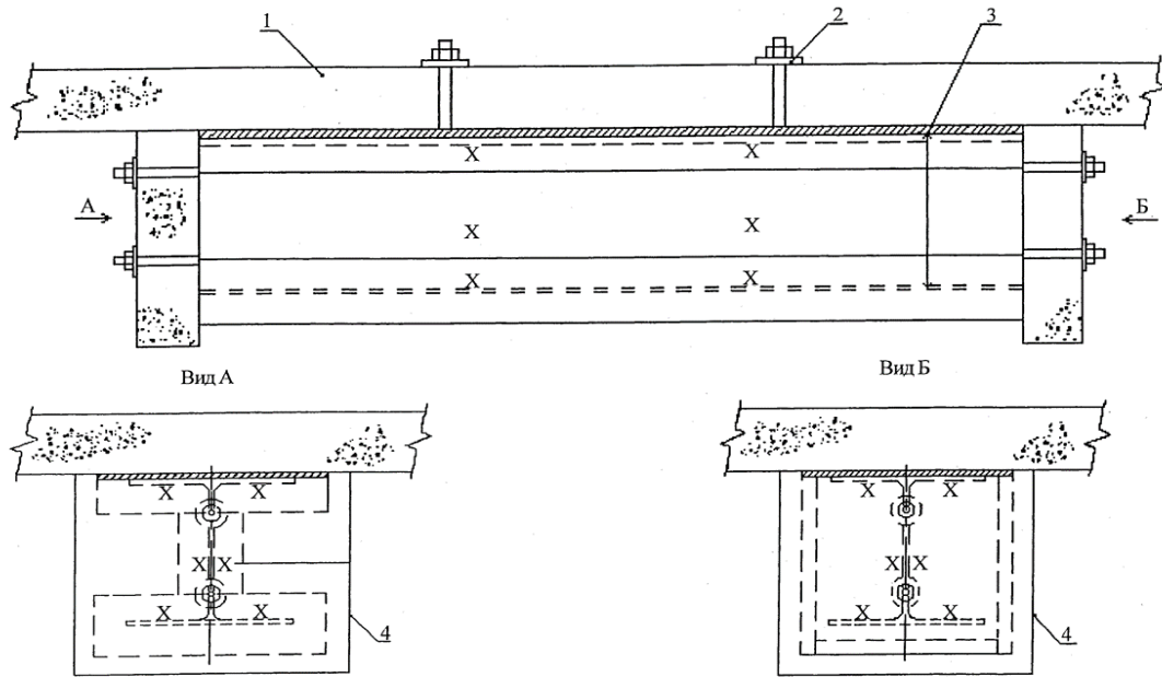
Рис. 1.12. Схема розміщення термопар для зразка ненавантаженої сталевій балки: 1 – плита печі верхня, 2 – кріпильні елементи, 3 – випробовуваний зразок, 4 – ізоляція кінців балки, х – термопара (вид А – із профільним перерізом, вид Б – коробчастий переріз)
