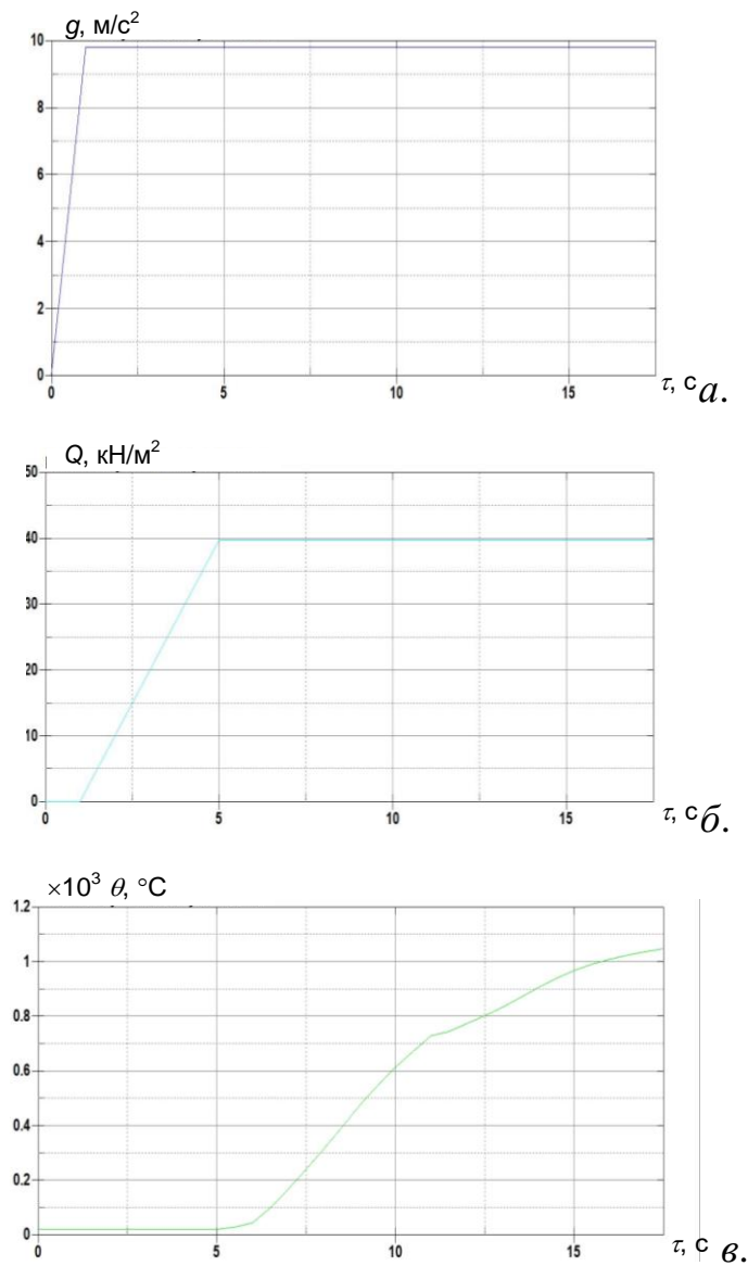
Рис. 4.14 Графіки залежності прикладених навантажень від часу: а – графік прискорення вільного падіння для врахування власної ваги; б – графік прикладення розподіленого навантаження; в – графік прикладення температурного навантаження
