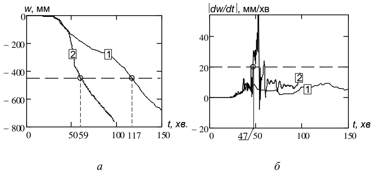
Рис. 5.4 Графіки зміни максимального прогину балки (а) та швидкості нарощування максимального прогину (б) залежно від часу впливу стандартного температурного режиму пожежі: 1 – для балки з мінераловатним вогнезахистом, що не втрачає своєї цілісності; 2 – для балки з мінераловатним вогнезахистом, що втрачає свою цілісність і вогнезахисну здатність.
