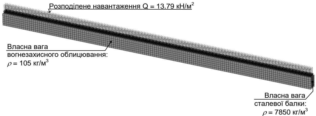
Рис. 4.13 Схема прикладання механічного навантаження до сталеві балки з вогнезахисним облицюванням із мінеральної вати
