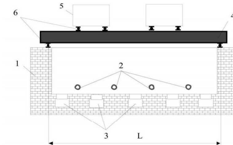
Рис. 1.10 Схема розміщення та кріплення горизонтального елемента у вогневій печі: 1 – стіни печі; 2 – пальники; 3 – канали для видалення продуктів згорання навантаження; 4 – зразок випробувань; 5 – навантаження; 6 – опори (шарнірні); L – довжина зразка, що зазнає вогневого впливу.
