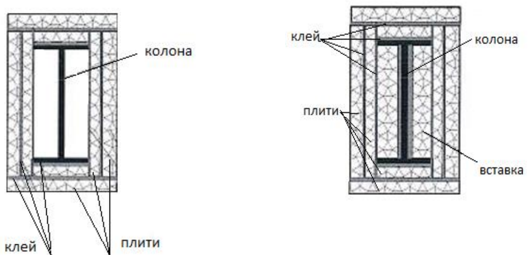
а – переріз зразків № 1, 2, 5, 6
