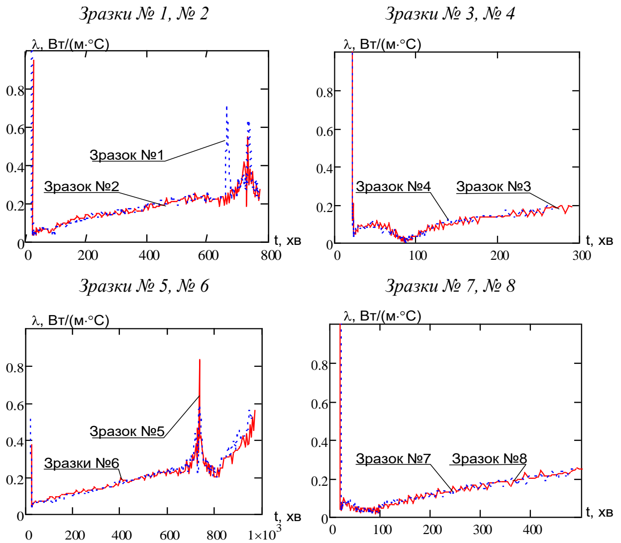
Рис. 3.11 Графіки залежностей коефіцієнта теплопровідності мінераловатного облицювання зразків фрагментів сталевих стержнів, згідно з температурою нагрівання фрагменту сталевих стержня
