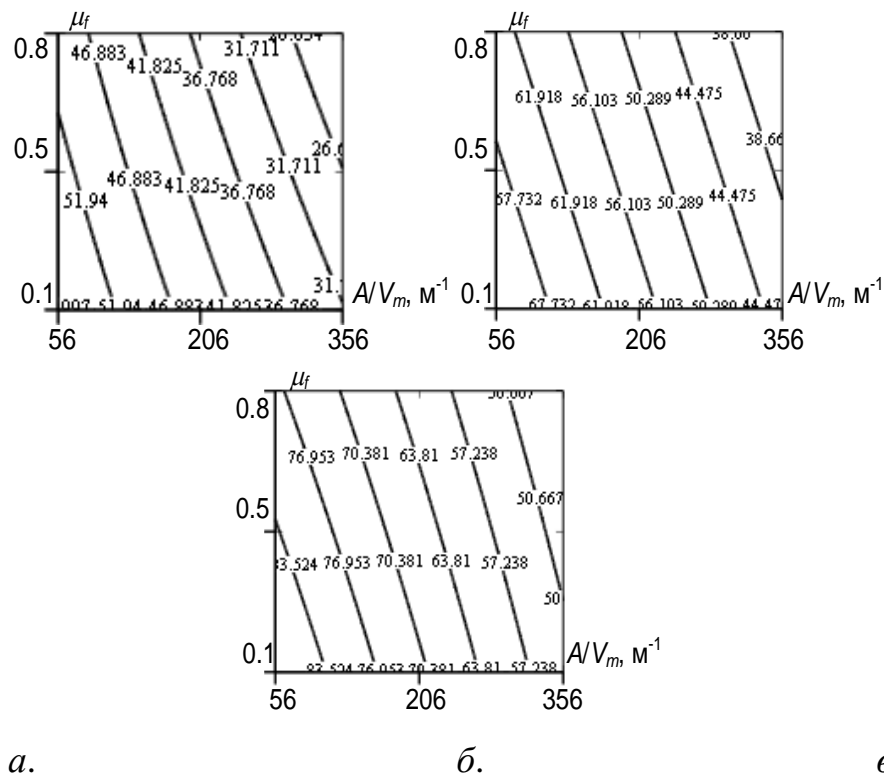
Рис. 5.7 Залежності часу відшарування вогнезахисного мінераловатного облицювання сталеві балки від коефіцієнта перерізу та коефіцієнта навантаження для різних значень його товщини: а – 25 мм; б – 50 мм; в – 75 мм.
