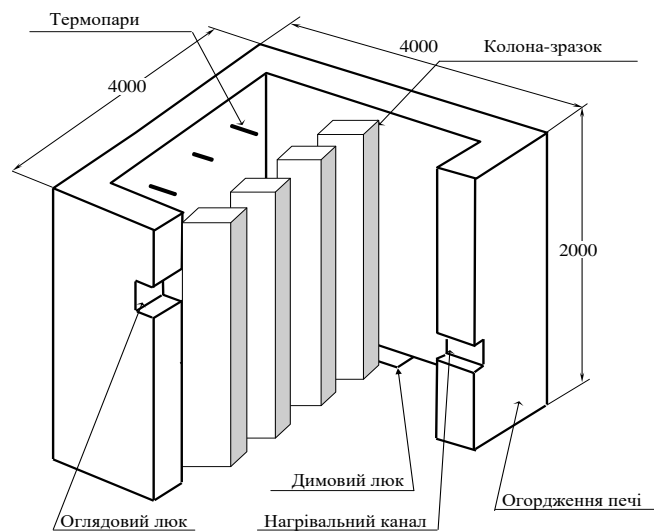
Рис. 2.2 Схема установки випробувальної вогневої печі
