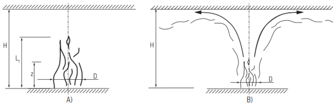
Рис. 1.6 Варіанти розвитку локалізованих пожеж
