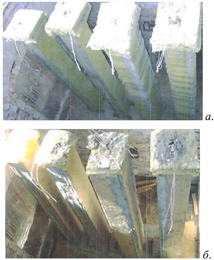
Рис. 3.1 Вигляд зразків № 1 – № 4: а – до початку випробувань; б – після випробувань
