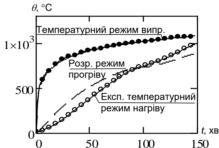
Рис. 3.9 Температурний режим нагрівання зразка 1, що отриманий розрахунковим та експериментальним способом
