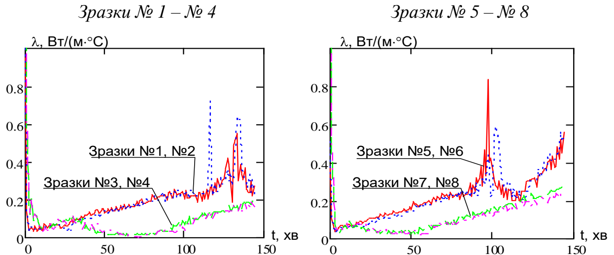
Рис. 3.10 Графіки залежностей коефіцієнта теплопровідності мінераловатного облицювання зразків фрагментів сталевих стержнів, відповідно до часу випробування
