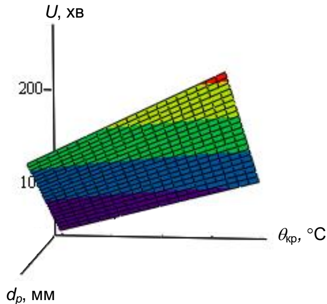
Рис. 3.7 Поверхня залежності часу досягнення критичної температури від найбільш значущих параметрів вогнезахисного елемента сталевій конструкції
