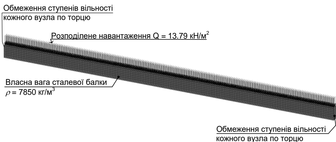
Рис. 5.3 Схема прикладання механічного навантаження до сталеві балки та умови закріплення
