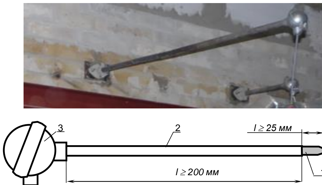
Рис. 2.4. Зовнішній вигляд та схема термопарі для вимірювання температури у вогневій камері печі: 1 – вимірювальний спай термопарі; 2 – захисний кожух; 3 – теплозахисна оболонка.
