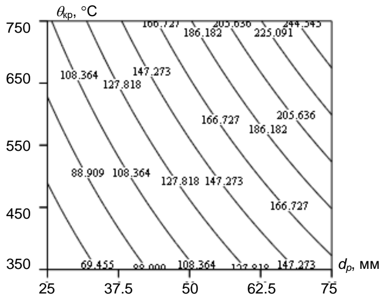
Рис. 3.8 Номограма для визначення межі вогнестійкості, що розрахована за умови досягнення критичної температури, з врахуванням товщини вогнезахисного мінераловатного облицювання
