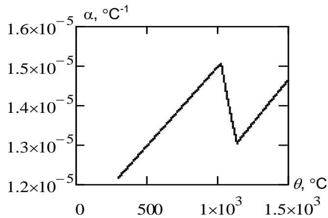
Рис. 4.9 Залежність коефіцієнта температурного розширення сталі від температури
