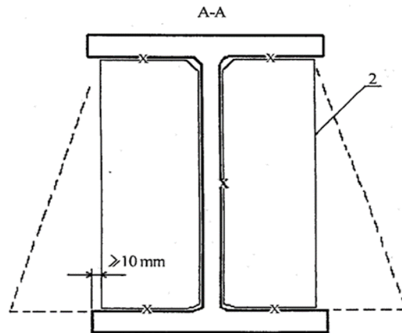
Рис. 1.13 Схема розміщення термопар для зразка навантаженої сталевій балки: 1 – навантаження, 2 – елементи жорсткості, виконані зі сталевих пластин, x – термопара (A-A – поперечний переріз балки з елементами жорсткості)
