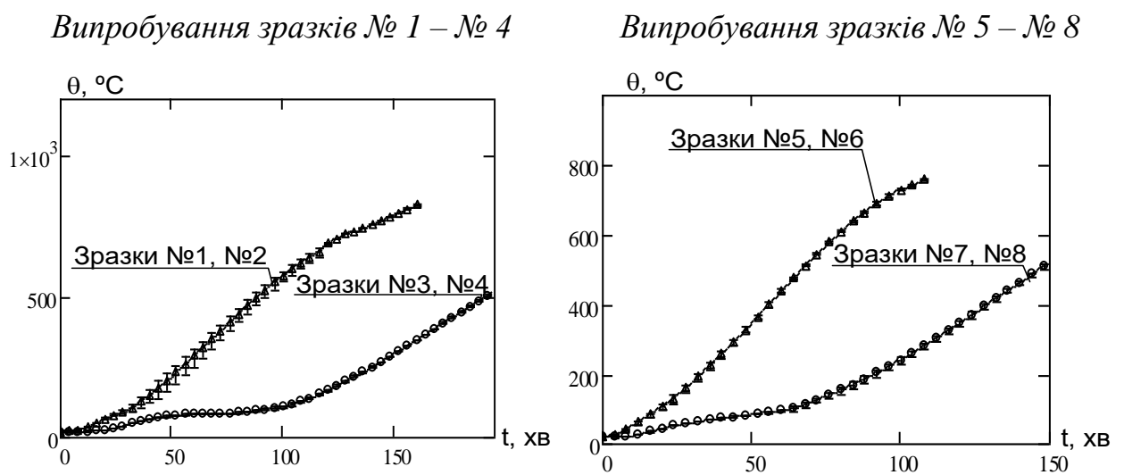
Рис. 3.5 Графіки показників середньої температури для кожного зразка за показниками з трьох термопар, встановлених на металевій поверхні залежно від часу випробувань
