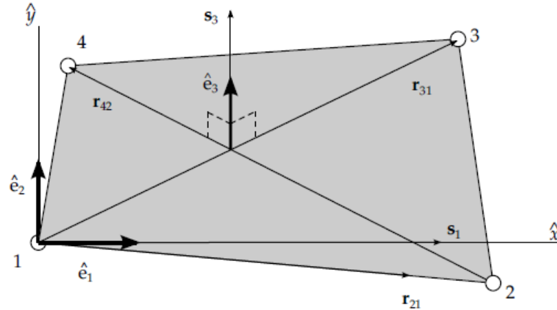
Рис. 4.7 Схема геометричних параметрів КЕ типу чотиривузлової оболонки Беличка – Цая
