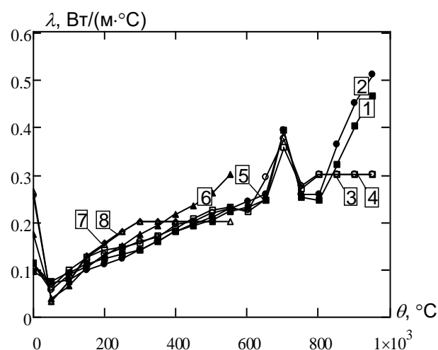
Рис. 3.12 Залежність усередненого значення коефіцієнта теплопровідності від температури зразків фрагментів сталевих стержнів із вогнезахисним облицюванням (1, 2, 3, ... – номери зразків)
