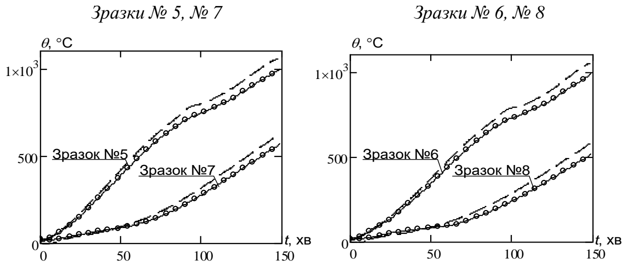
Рис. 3.14 Графіки температурних режимів прогрівання залежностей сталевих елементів стержнів із мінераловатним вогнезахисним облицюванням: \circ-\circ-\circ - експериментальні дані; -\ - - - розрахункові дані.
