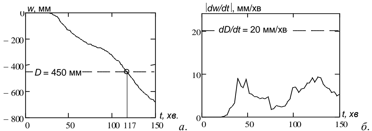
Рис. 4.18 Графіки зміни максимального прогину балки (а) та швидкості нарощування максимального прогину (б), залежно від часу впливу стандартного температурного режиму пожежі
