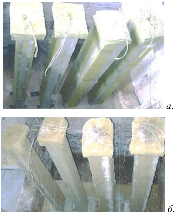
Рис. 3.2 Вигляд зразків № 5 – № 8: а – до початку випробувань; б – після випробувань
