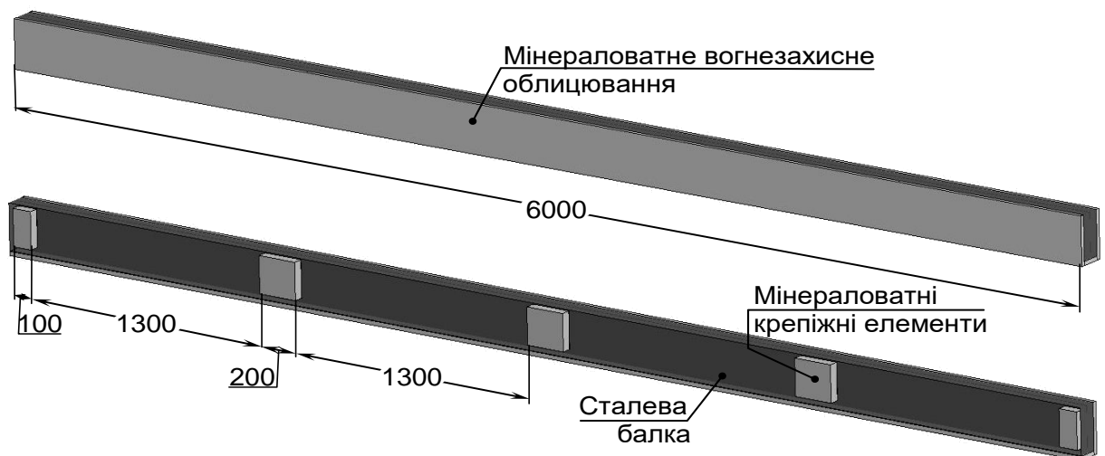
Рис. 4.11 Конструктивна схема сталевій балки з вогнезахисним облицюванням із мінеральної вати
