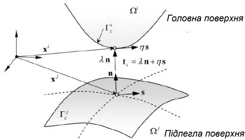
Рис. 4.5 Схема визначення геометричних параметрів контакту
