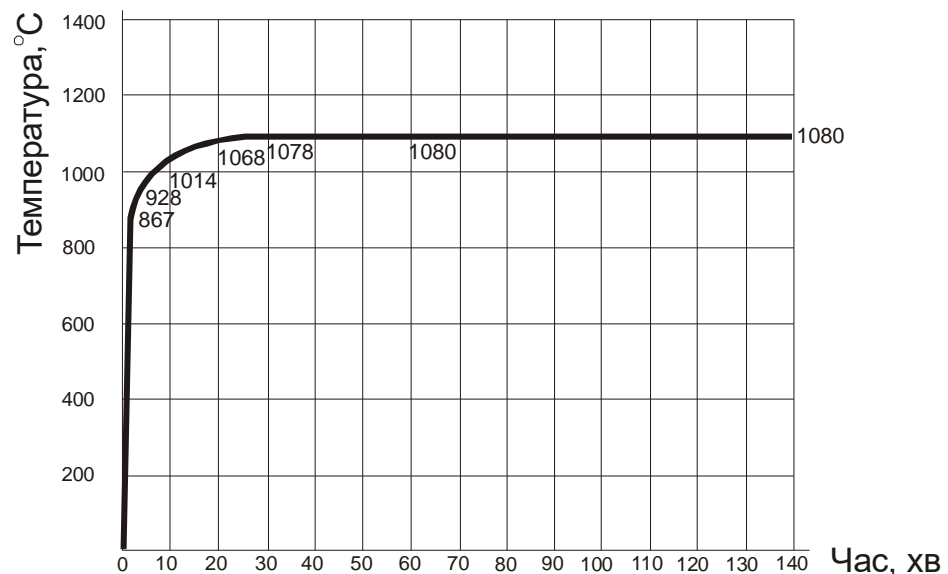
Рис. 1.4. Графік температура-час режиму вуглеводневої пожежі (відношення зростання температури до часу)
