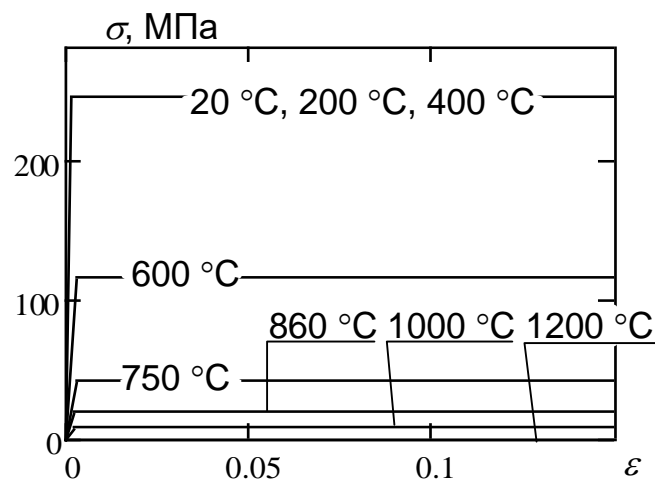
Рис. 4.10 Діаграми деформування сталі С 245 залежно від температури нагрівання
