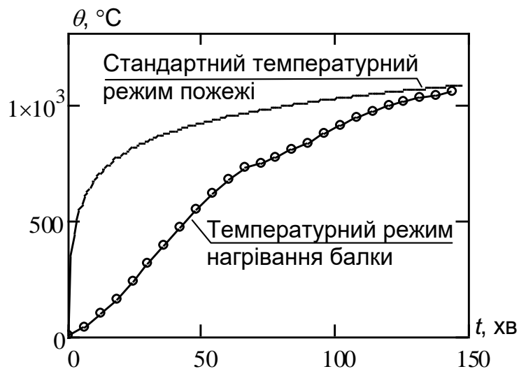
Рис. 4.2 Температурний режим нагрівання сталеві балки з мінераловатним вогнезахисним облицюванням за умов впливу стандартного температурного режиму пожежі
