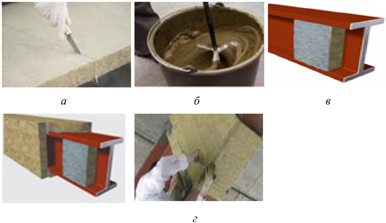
Рис. 2.6 Етапи виготовлення експериментальних зразків: а – розрізання теплоізоляційних плит за розмірами й товщиною; б – приготування клеєвої суміші «Ceresit CM-17»; в – закріплення мінераловатних вставок клеєвою сумішшю; г – закріплення мінераловатного облицювання клеєвою сумішшю.
