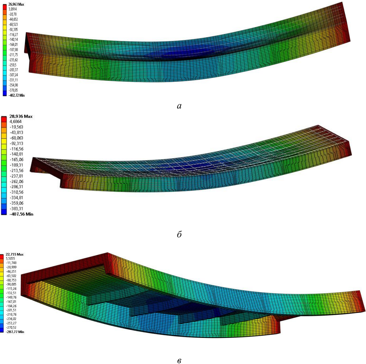
Рисунок 5. Прогини залізобетонній ребристий плити при пожежі за рівними навантаження (а - 2,55 кПа; б - 3,57кПа; в - 5,1 кПа)
