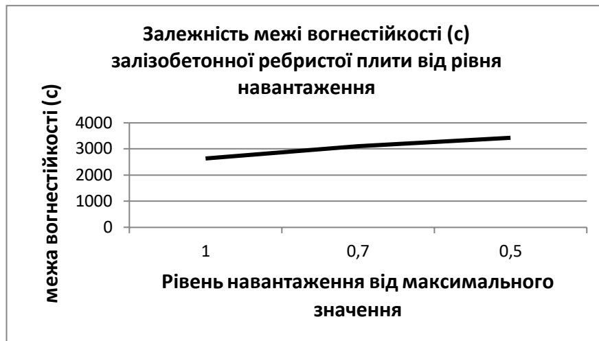
Рисунок 7 – Залежність між показниками вогнестійкості та рівнем механічного навантаження залізобетонній ребристій плити
