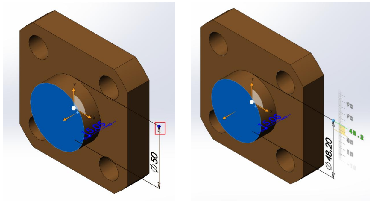
Рисунок 6.12 – Корегування розмірів за допомогою Instant 3D
