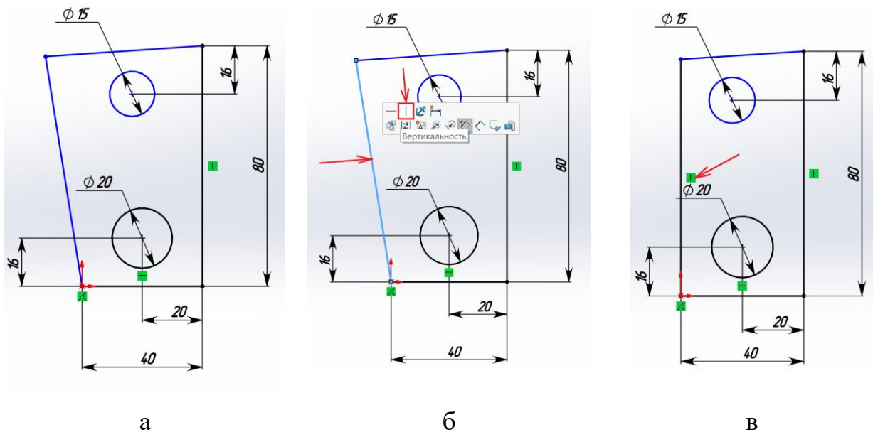
Рисунок 2.17 – Додавання взаємозв'язку «Вертикальність» I
