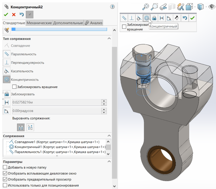
Рисунок 5.15 – Умова сполучення «Концентричність»
