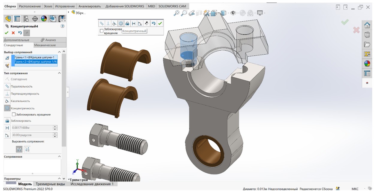
Рисунок 5.11 – Умова сполучення «Концентричність»
