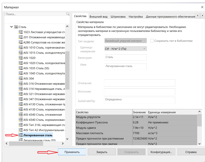
Рисунок 3.17 – Вибір матеріалу виготовлення деталі
