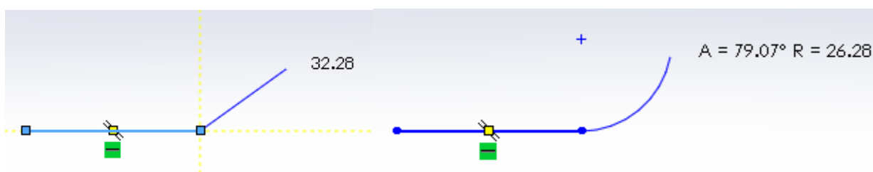
Рисунок 2.8 – Автоматичний перехід від лінії до дотичної дуги
