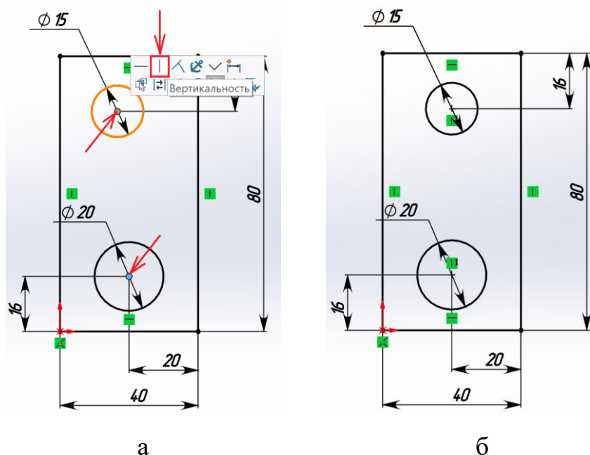
Рисунок 2.19 – Додавання взаємозв'язку «Вертикальність»
