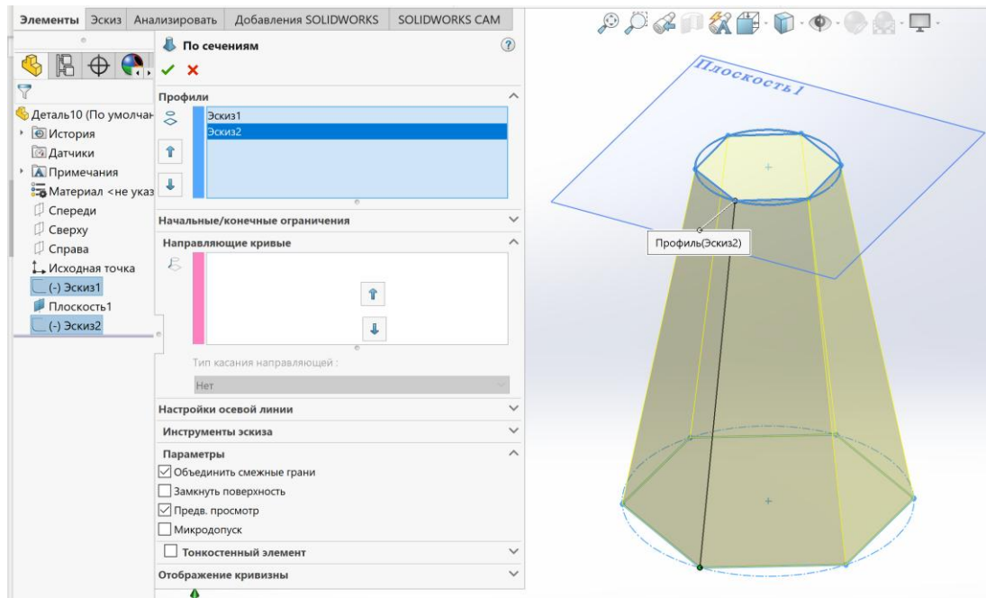
Рисунок 3.13 – Побудова елемента «Бобишка/основа по перетинах»
