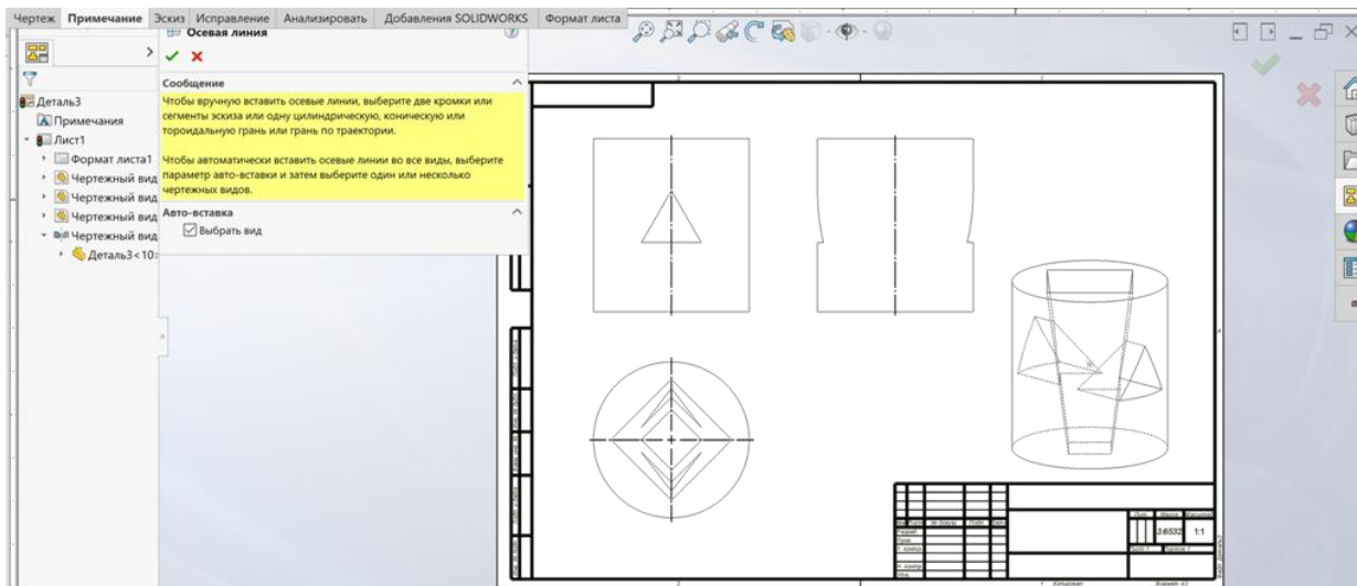
Рисунок 4.8 – Нанесення осевих ліній
