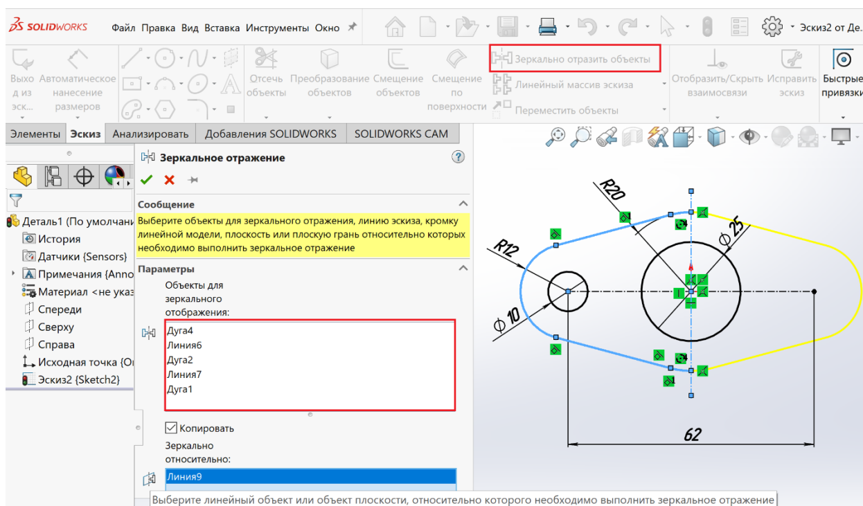
Рисунок 2.26 – Дзеркальне відображення об'єктів
