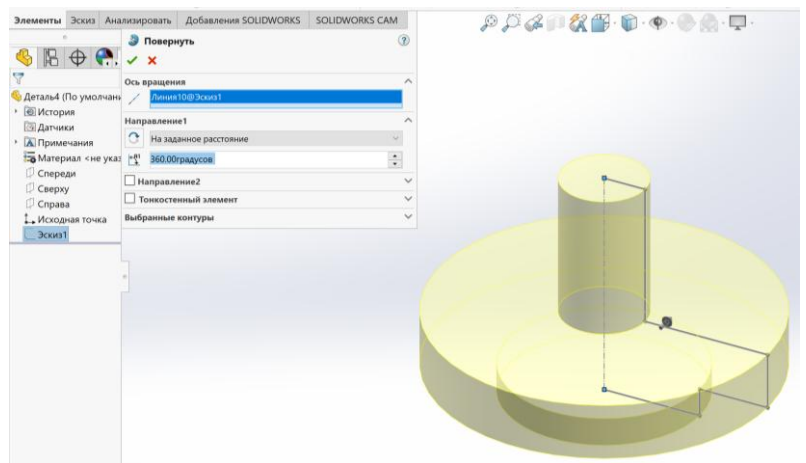
Рисунок 3.7 – Інструмент «Повернута бобишка»
