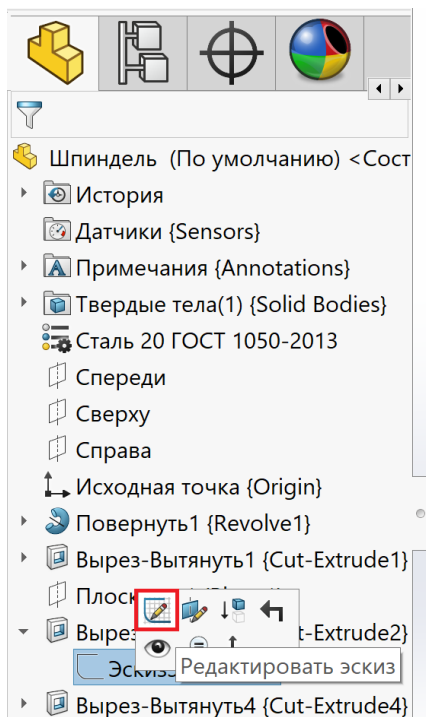
Рисунок 3.19 – Редагування існуючого ескізу з Древа конструювання
