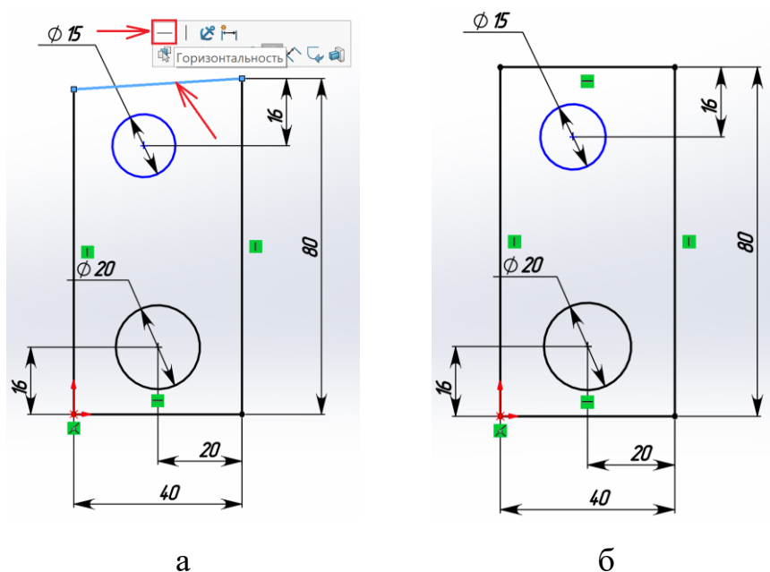
Рисунок 2.18 – Додавання взаємозв'язку «Горизонтальність» —
