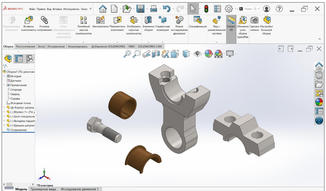
Рисунок 5.4 – Компоненты збірки
