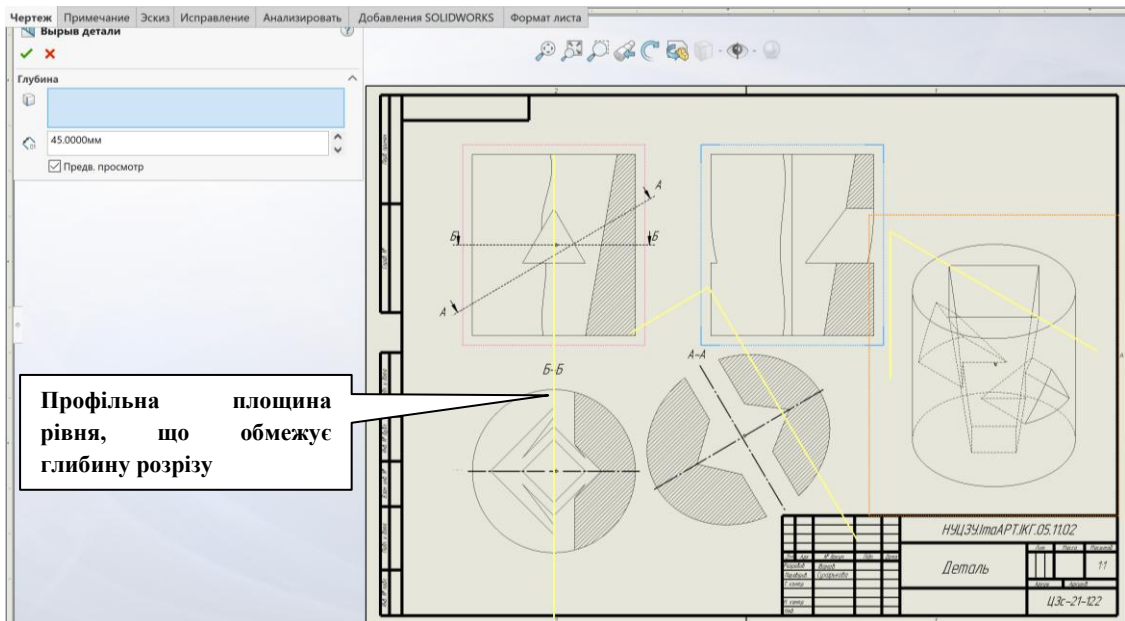
Рисунок 4.17 – Побудова профільного розрізу
