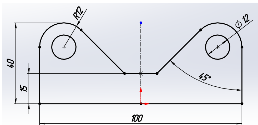
Рисунок 6.6 – Приклад симетричної деталі
