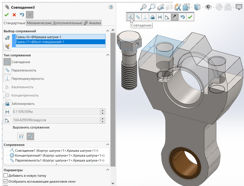
Рисунок 5.14 – Умова сполучення «Збіг»
