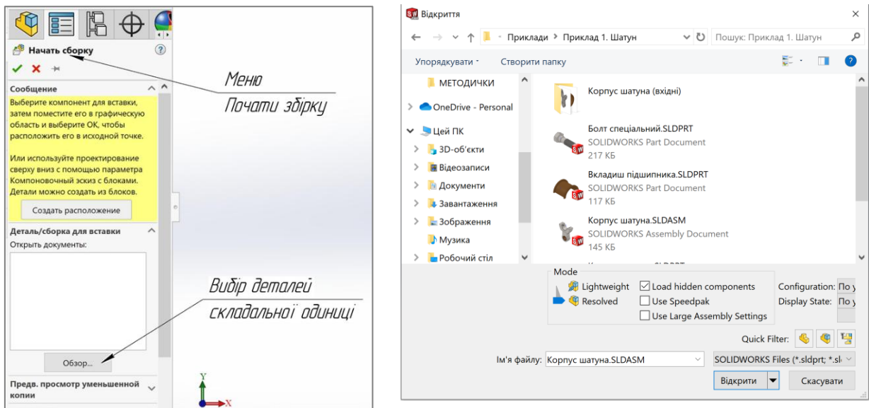
Рисунок 5.3 – Додавання компонентів збірки
