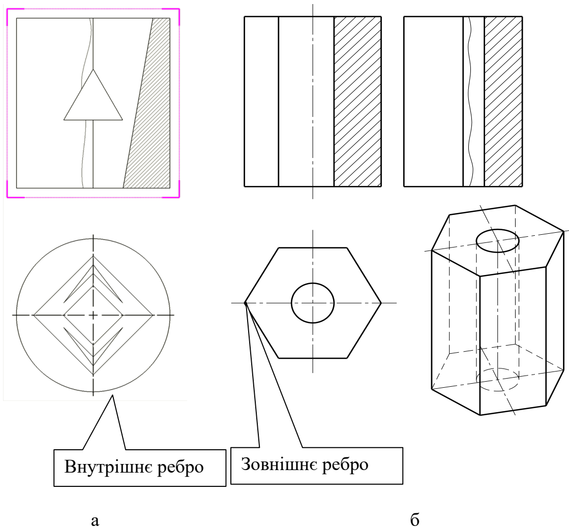
Рисунок 4.11 – Розмежування виду та розрізу в залежності від розташування ребра
