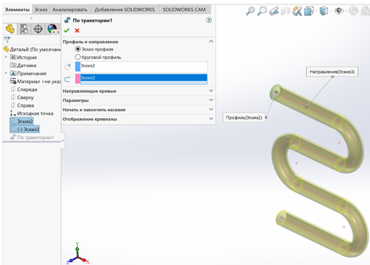
Рисунок 3.9 – Элемент «Бобишка/основа по траектории»
