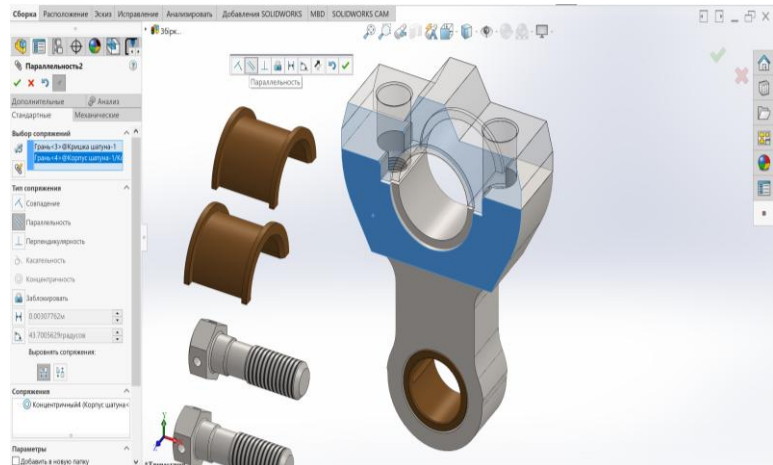
Рисунок 5.13 – Умова сполучення «Паралельність»
