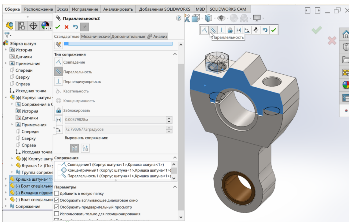
Рисунок 5.16 – Умова сполучення «Паралельність»
