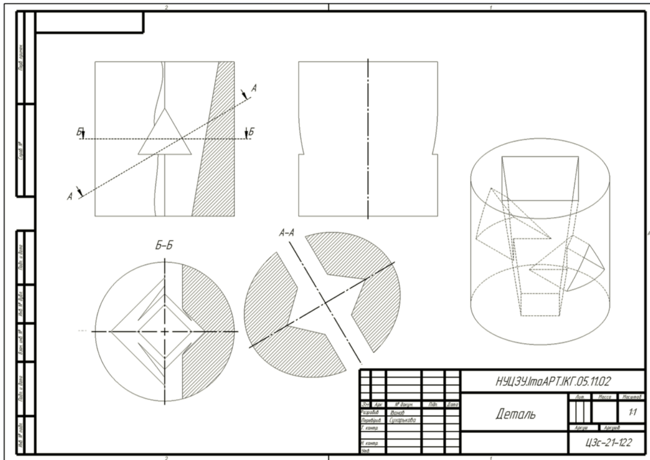
Рисунок 4.16 – Позначення горизонтального розрізу
