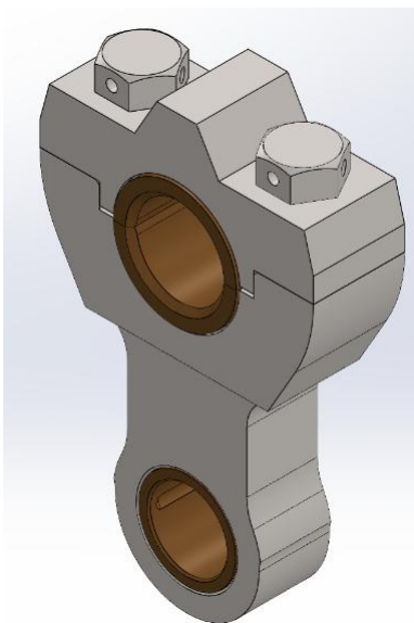
Рисунок 5.1 – Шатун
