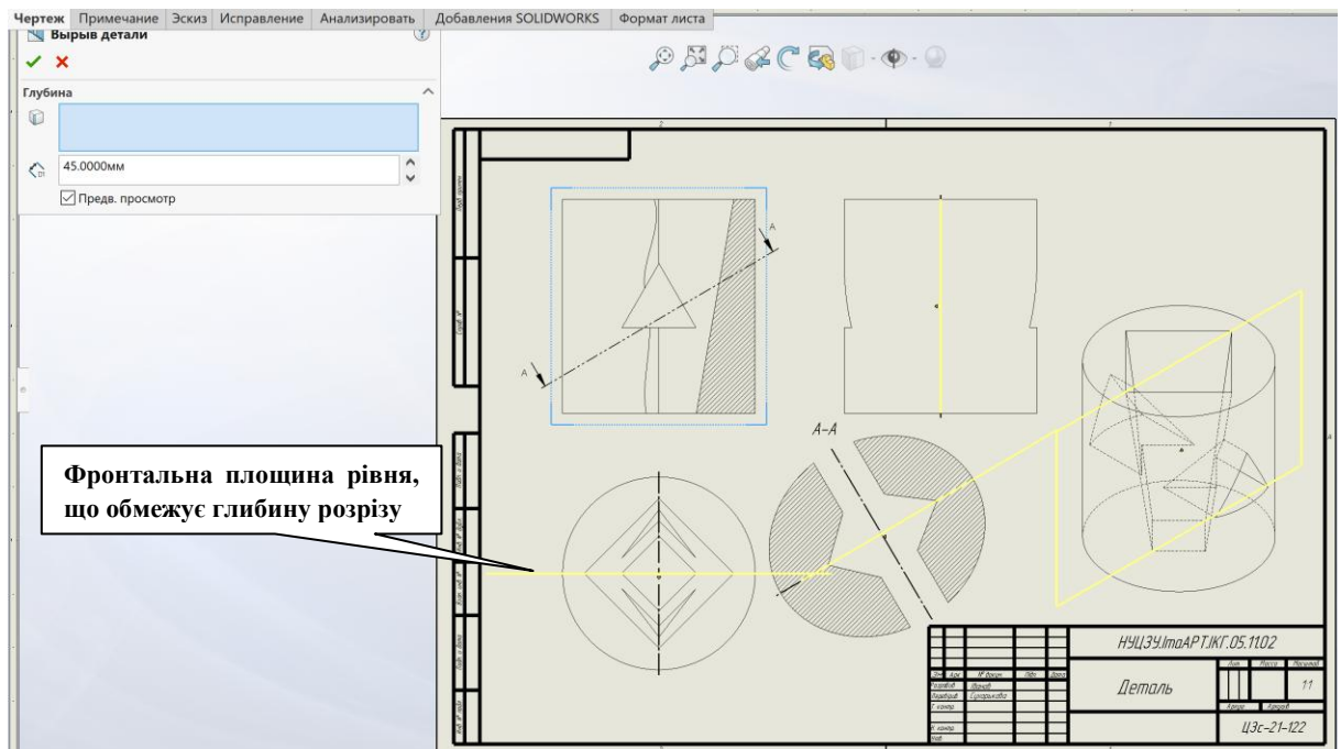
Рисунок 4.13 – Суміщення половини виду Спереду з фронтальним розрізом
