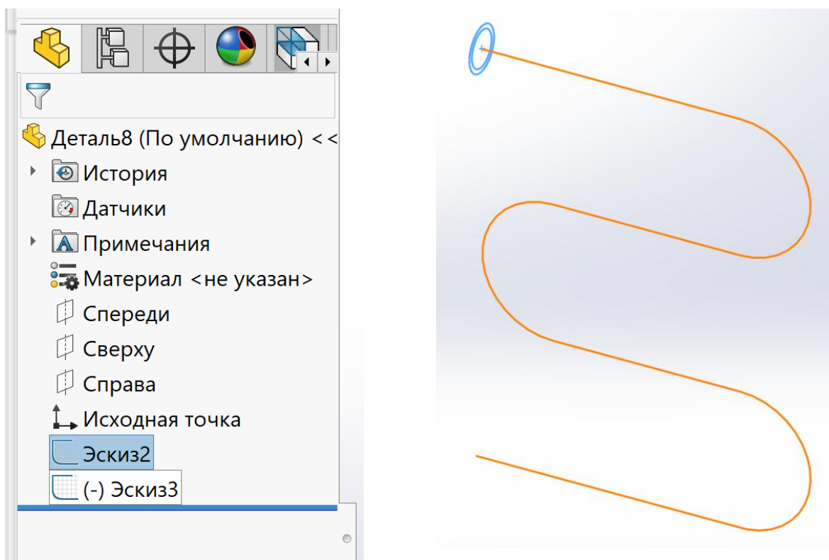
Рисунок 3.8 – Ескізи для елемента «Бобишка/основа по траєкторії»
