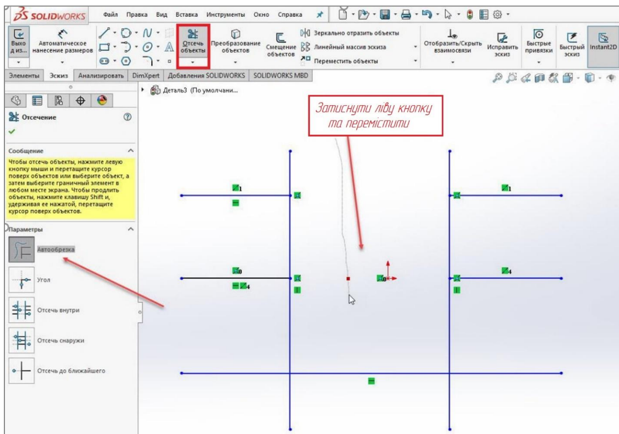
Рисунок 2.22 – Видалення частин об'єктів за допомогою автообрізки
