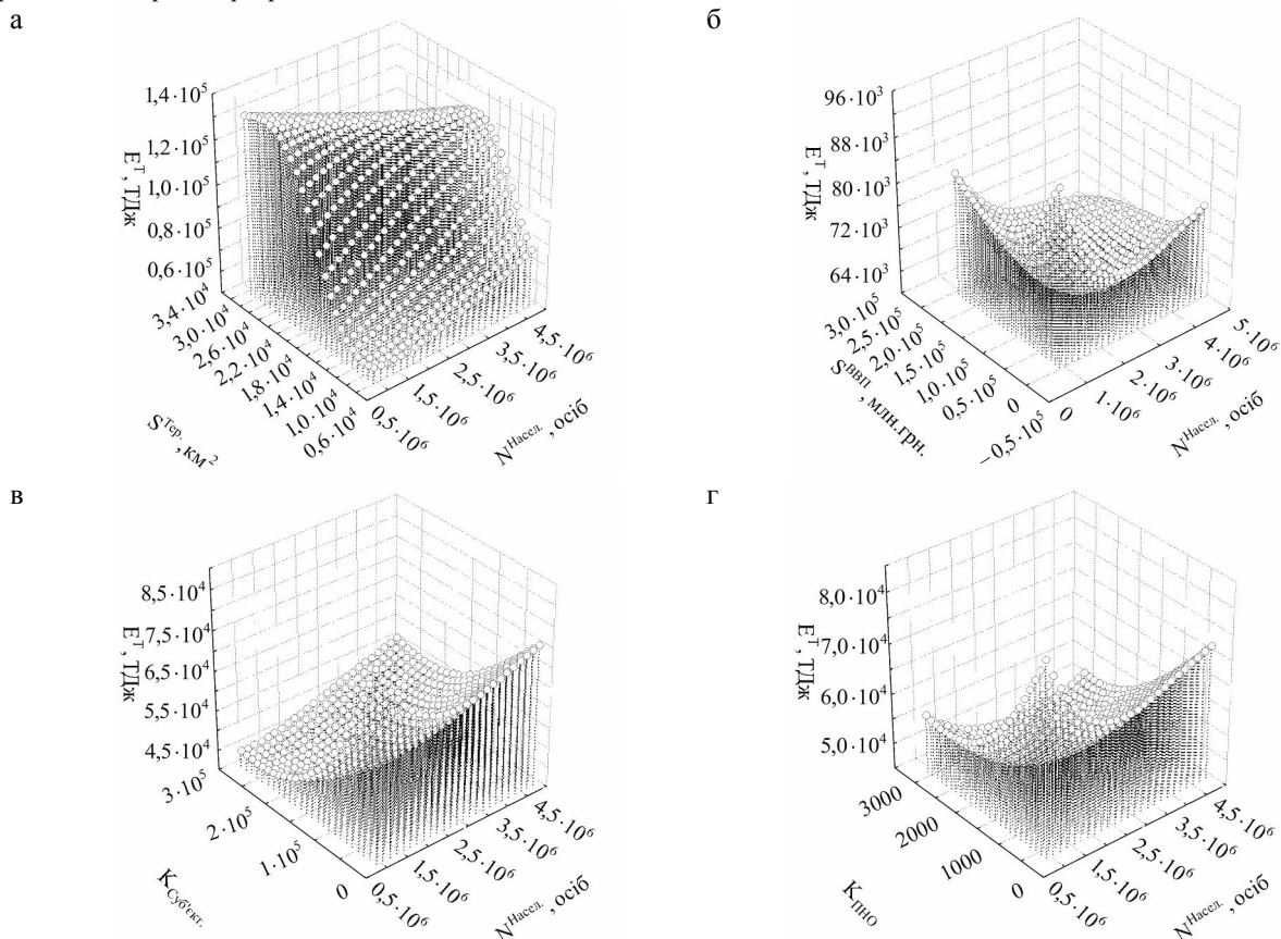
Рис. 5. Приклади поверхонь відгуку мережею БШП 13:13-30-1:1 за енергією техногенного походження від основних показників повсякденного функціонування: а – чисельності наявного населення та площі території; б – чисельності наявного населення та об'єму валового внутрішнього продукту; в – чисельності наявного населення та кількості суб'єктів Єдиного державного реєстру підприємств та організацій України; г – чисельності наявного населення та кількості потенційно небезпечних об'єктів
