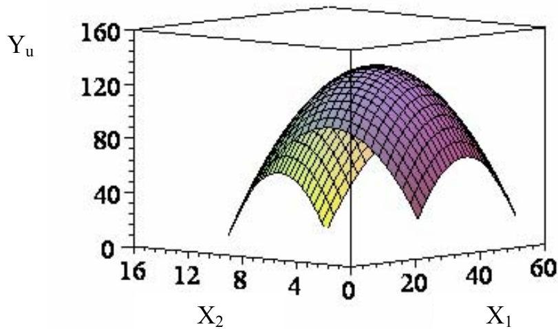
Рисунок 1 – Зависимость отклика аналитического сигнала насыщения ПД ГПИ от тока и количества витков нагревателя
