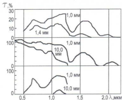
Рис. 1. Отражательная способность человеческой кожи /
