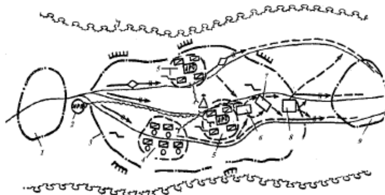
1 – район очікування; 2 – контрольно-розподільний пост; 3 – межа розгортання майданчиків спеціальної обробки; 4 – майданчик обробки за допомогою дегазаційних комплектів; 5 – майданчик обробки АРС; 6 – майданчик обробки обладнання; 7 – майданчик обробки засобів індивідуального захисту; 8 – майданчик заміни забрудненого обмундирування; 9 – район збору.
